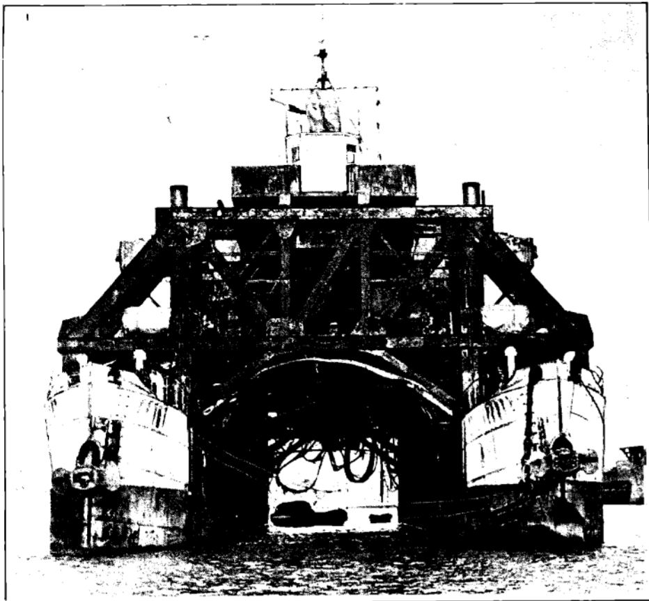
Aquí vemos al "rescatador de submarinos inventado por un ingeniero alemán, y con el cual se trata de recuperar el submarino inglés M-1, que se ha hundido en el centro del Canal de la Mancha.
